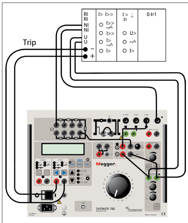
使用SVERKER 780测试吸合和释放
